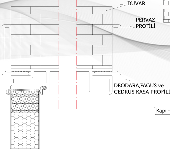
Kapı - Kasa Bağlantı Detay Üst
