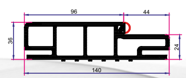
140mm KAPI KASA
